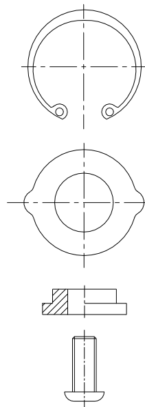
Type 2 Retainer Assembly C06.DDD.000
